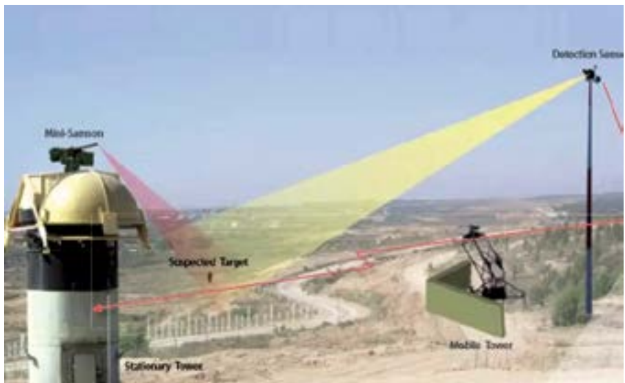
מערכת "רואה יורה". לאחר זיהוי אויב בשטח, התצפיתניות מפעילות את אמצעי הירי
